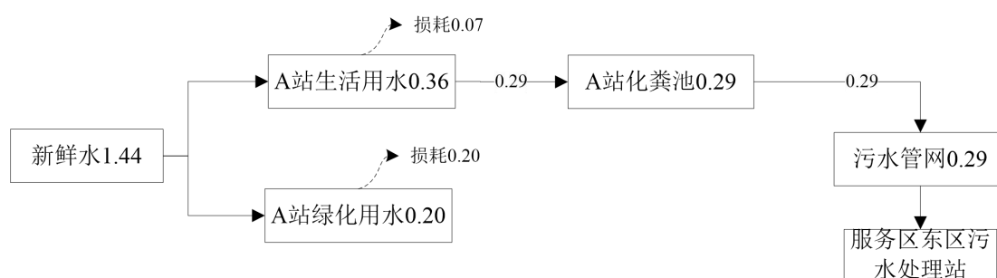
图 2-1 验收阶段工程实际用水平衡图 单位：m 3 /d
