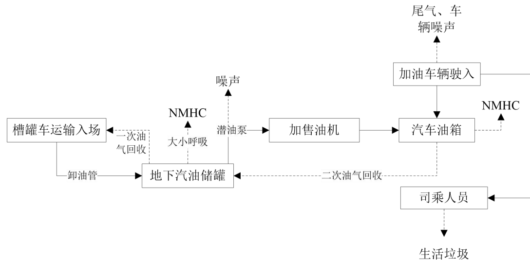
图 2-2 运营期汽油加油流程及产污环节图
