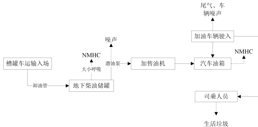
图 2-3 运营期柴油加油工艺流程及产污环节图
