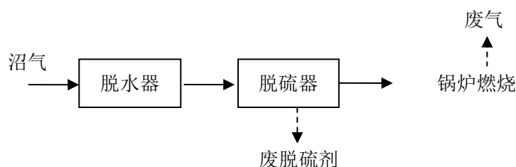
图 3.2-4 沼气利用流程及产物环节图
