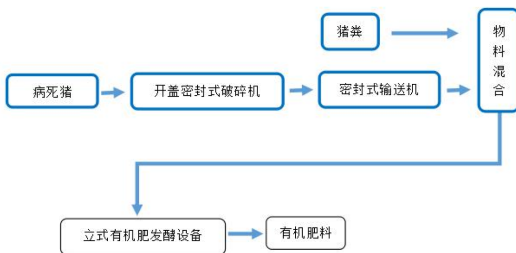
图 3.2-5 病死猪及胎盘处理工艺流程图
