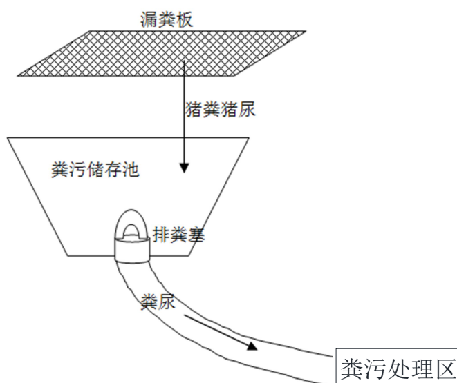
图 3.2-2 本项目清粪工艺示意图
