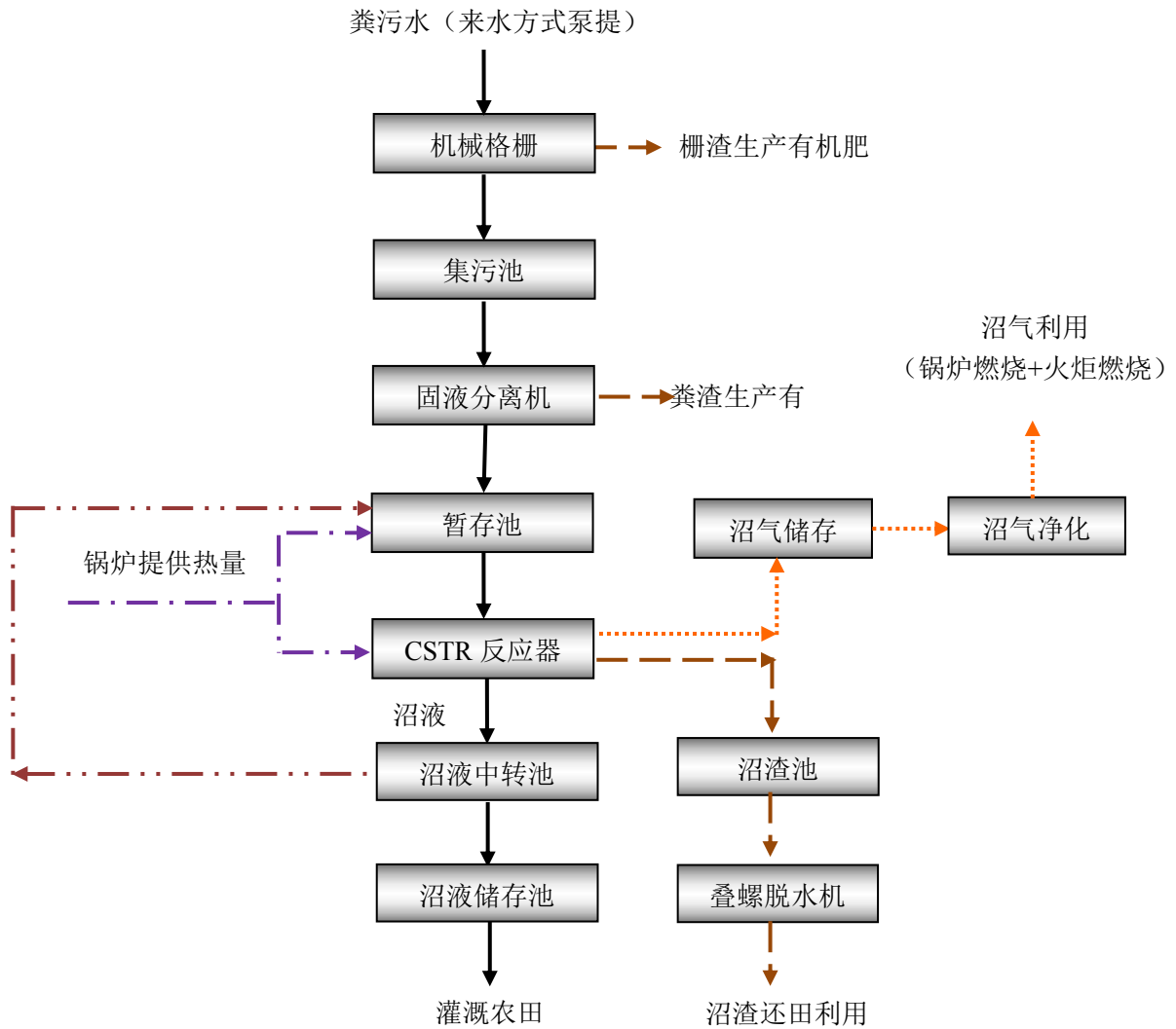
图 3.2-3 项目粪污水处理工艺流程图
