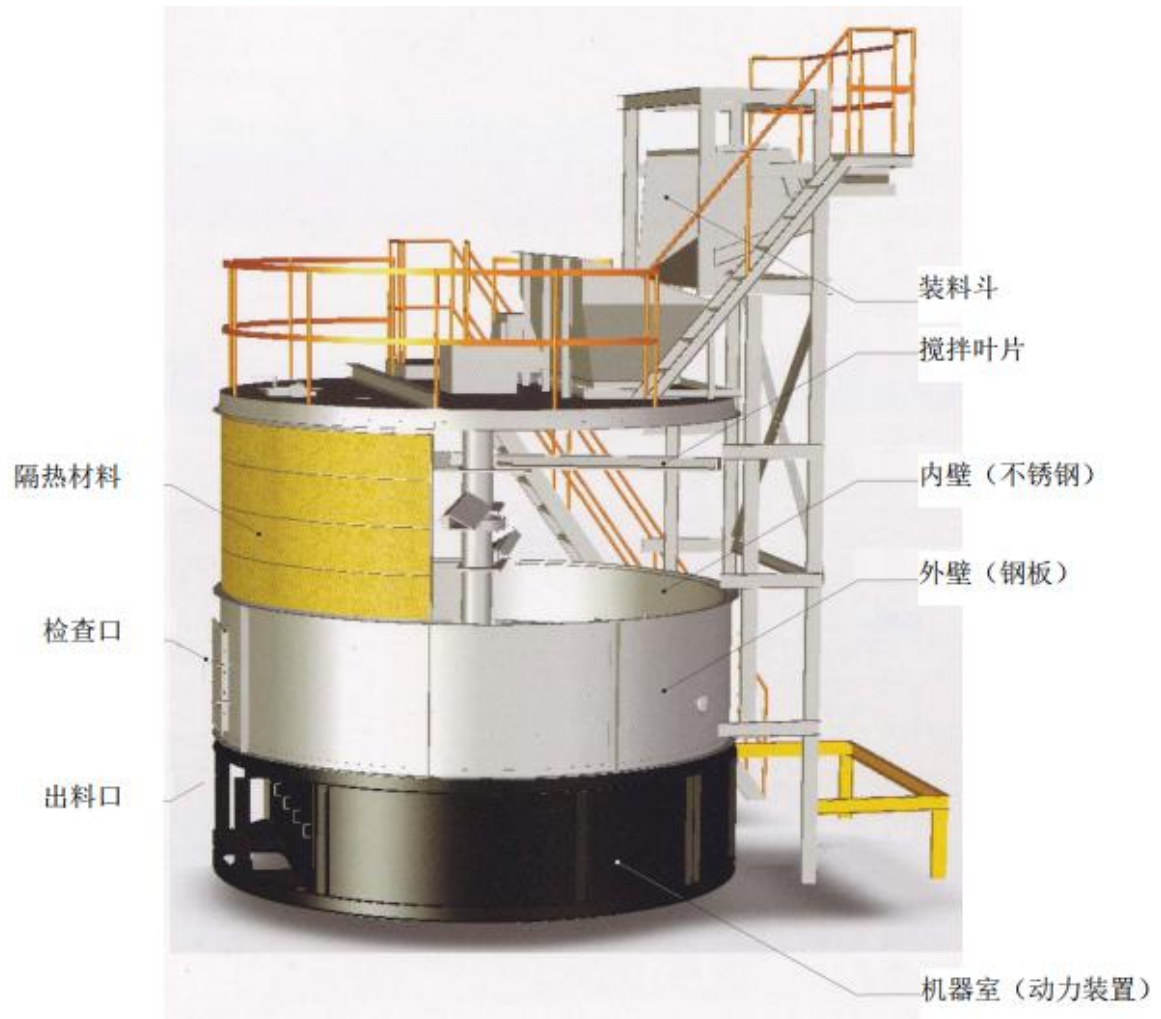
图6.2-1 立式发酵罐构造图
